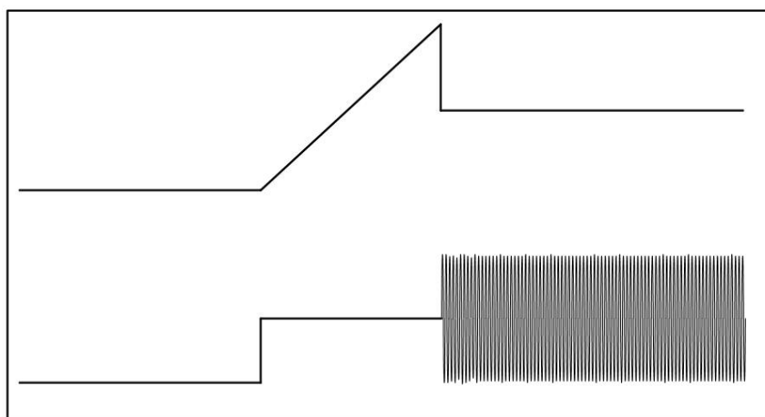
图 3：VCC 启动
